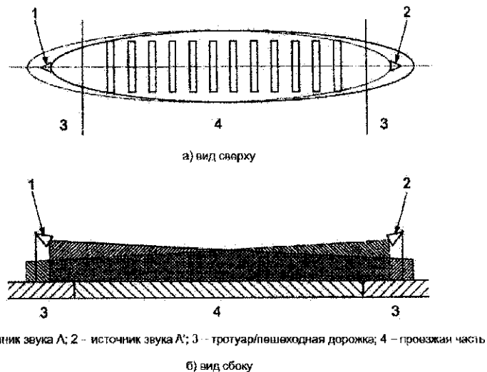
Рисунок 1 – Зона слышимости звукового сигнала переменной частоты (вид сверху, вид сбоку)
